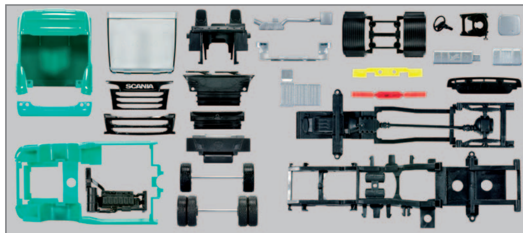
Schnappbautechnik: Die 31 Einzelteile des Scania Fahrerhauses sind so exakt konstruiert, dass sie von den Herpa-Mitarbeitern ohne Kleber zusammengesteckt werden können. / Snap Construction: The 31 items of the Scania cab are designed precisely, so that they can be put together from Herpa employees without glue.
