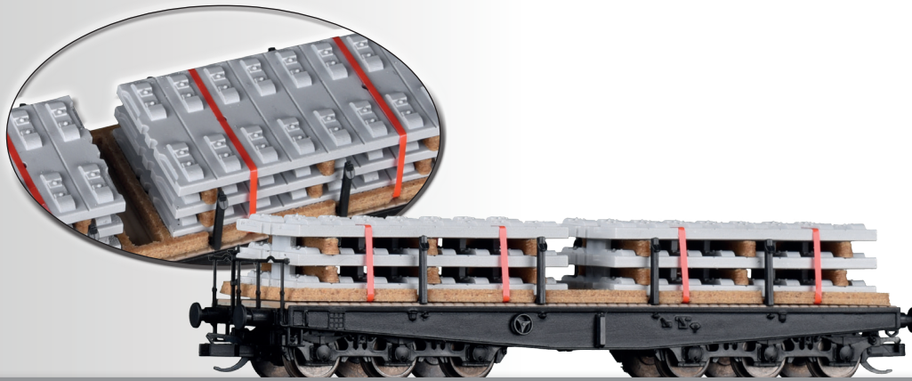
Schwerlastwagen Sammp 705 der DB AG, beladen mit Betonteilen „Feste Fahrbahn Bögl“
