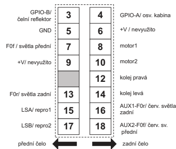
zapojení pinů Plux16, deska DPS
